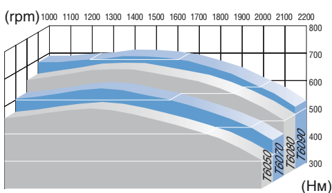
Кривая крутящего момента
